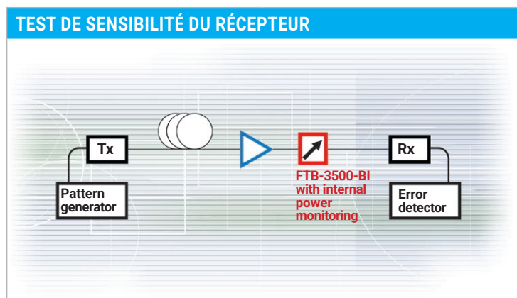
Configuration typique de la sensibilité du récepteur
