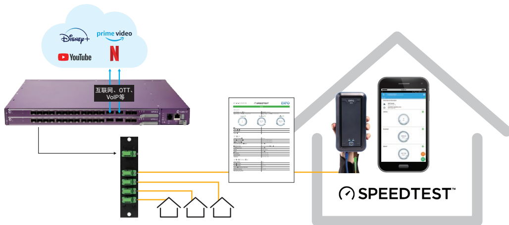
图3: 在XGS-PON上进行Speedtest测试
