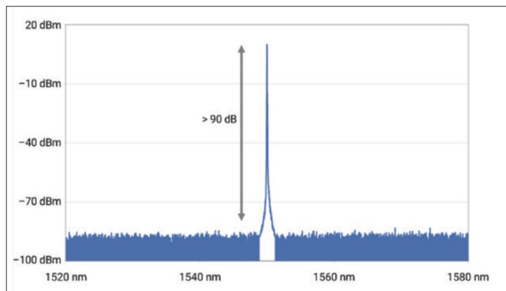
Figure 2. Puissance élevée et plage dynamique étendue.
