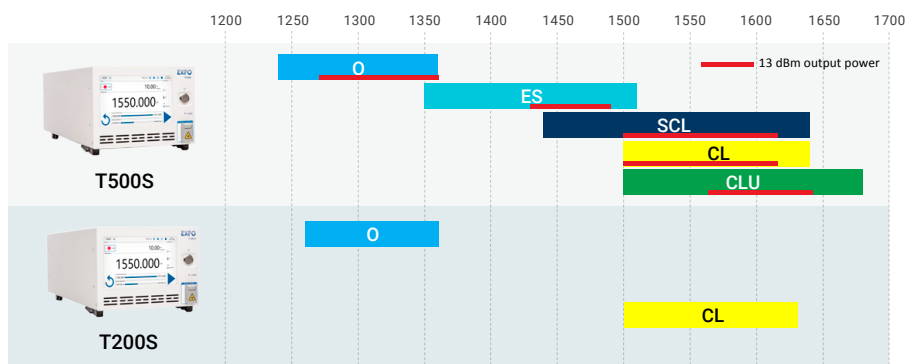
Figure 1. Couverture spectrale des différents modèles T200S-T500S.
