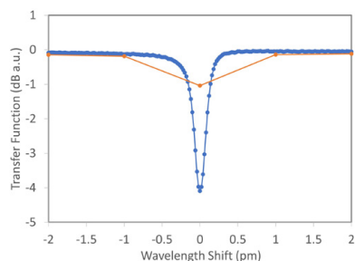
Figure 3. Mesure par résonateur en anneau avec une résolution de 20 fm et une résolution de 1 pm.
