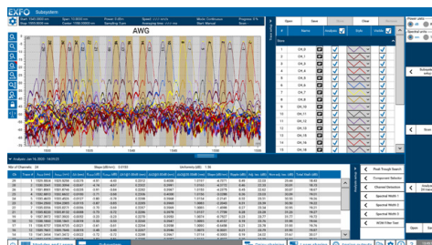
Figure 4. Écran de mesure.
