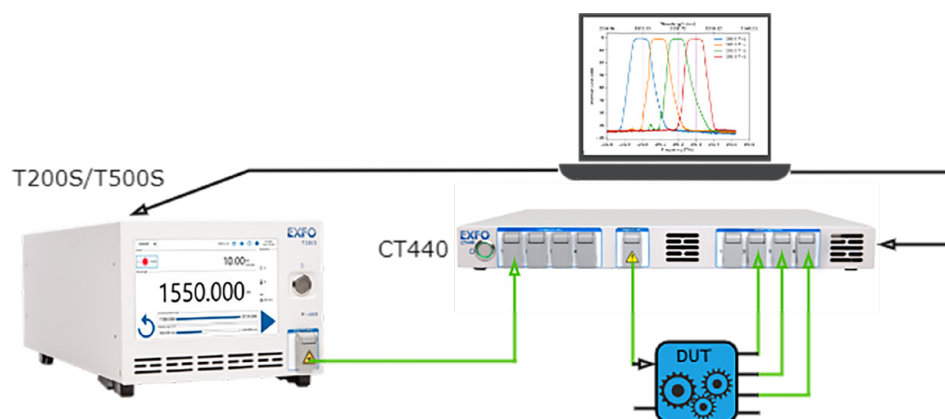
Figure 5. Configuration de mesure type utilisant le testeur de composants CT440 avec un laser accordable T200S/T500S.
